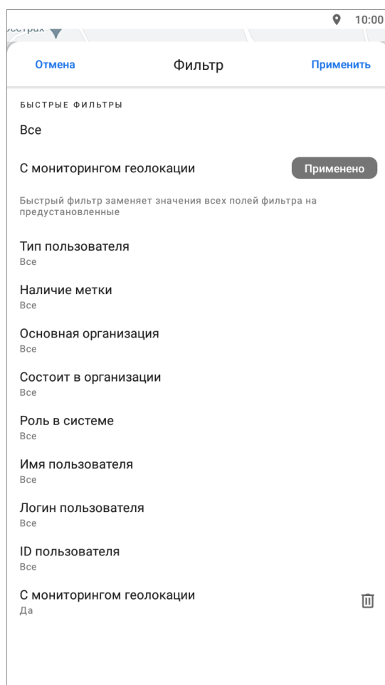
Рис. 2.95: Окно расширенного фильтра сотрудников
