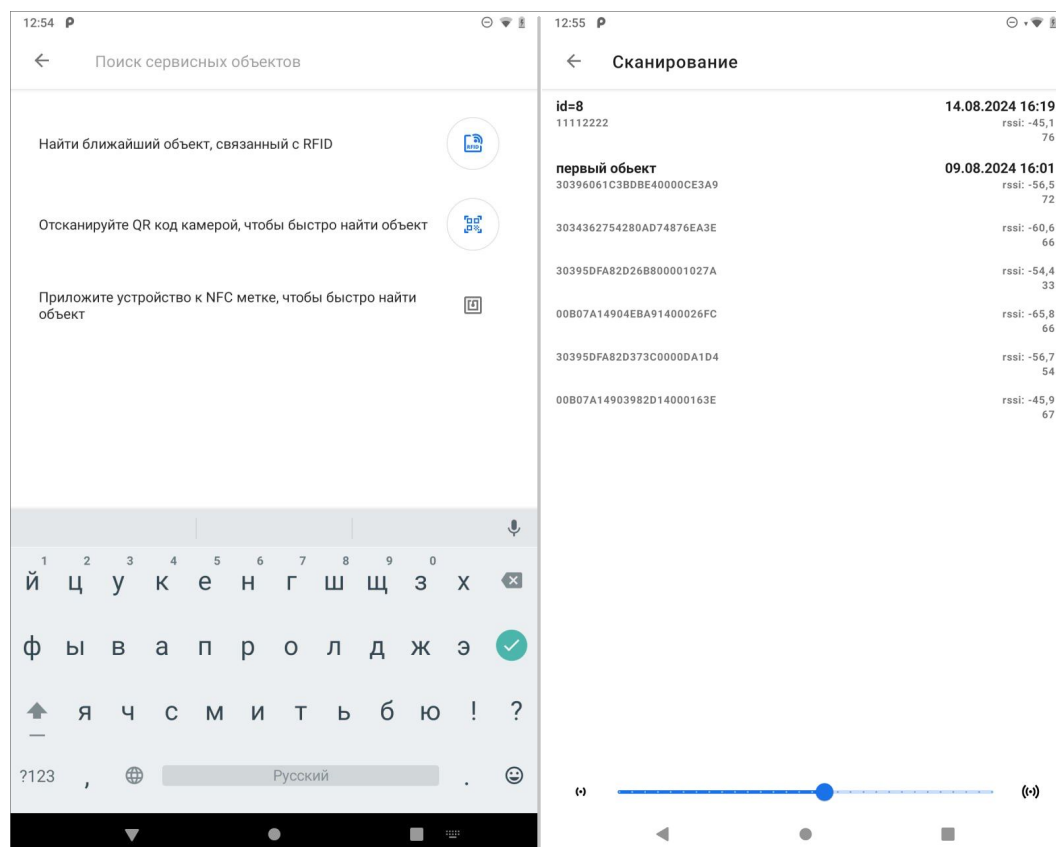
Рис. 2.124: Поиск объектов, связанных с RFID
