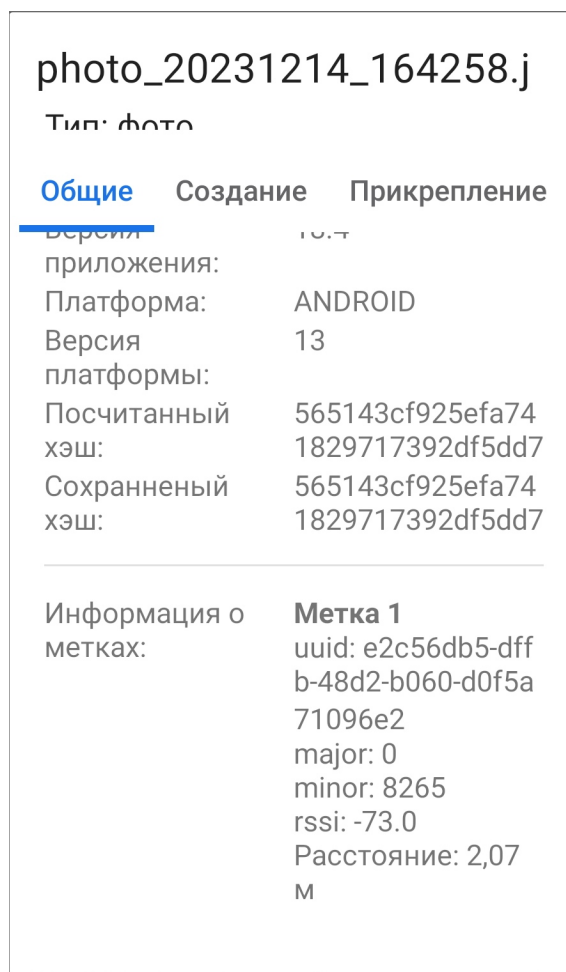
Рис. 2.41: Информации о BLE-метках в фотографии
