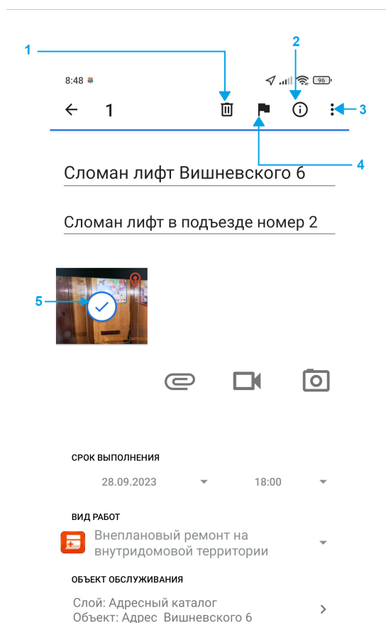
Рис. 2.39: Схема окна «Создания задания» в режиме работы с медиафайлами (1 - удаление вложения, 2 - информация о файле, 3 - меню окна, 4 - стикеры, 5 - выделенный файл)
