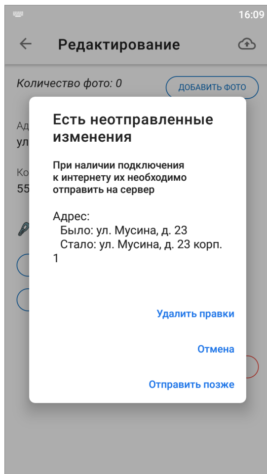
Рис. 2.85: Отправка или отмена изменений
