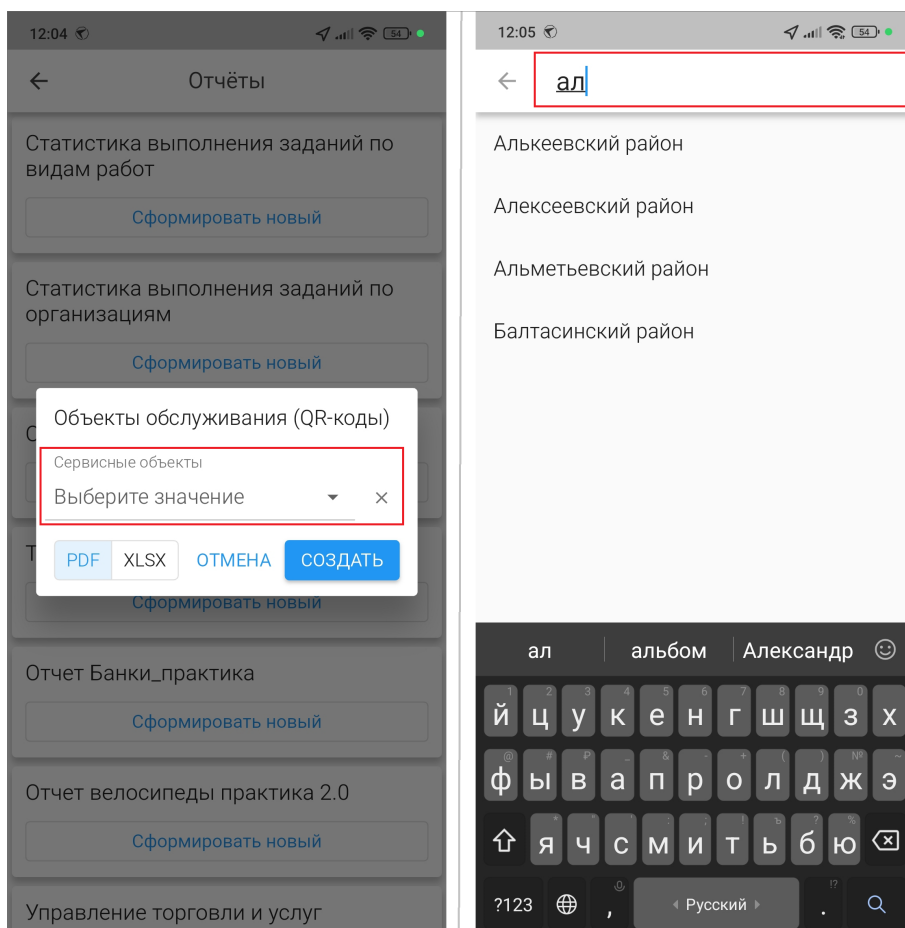
Рис. 2.114: Поиск среди значений параметров
